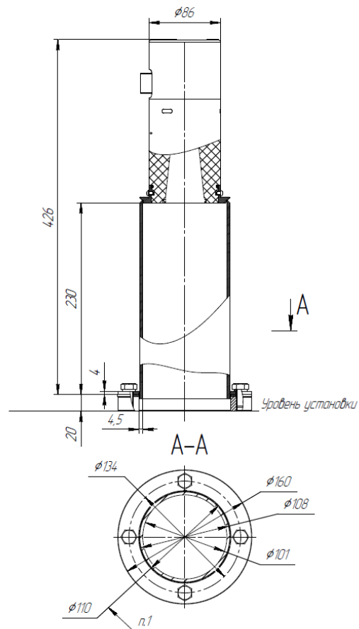
Рисунок 9. Габаритные и присоединительные размеры У-150 с герметичной стойкой
