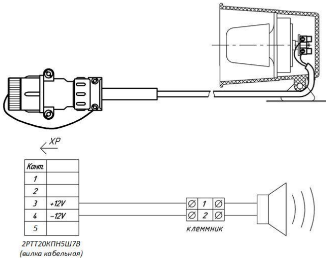
Схема подключения оповещателя к У-150Д
