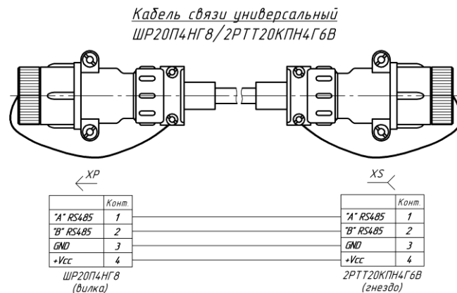
Рисунок 11. Кабель связи универсальный ШР20/ШР20
