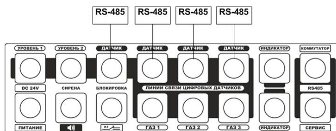
Рисунок 12. Разъемы МУ-150/МУ-150Е/МК-140 для подключения У-150
