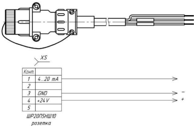
Кабель 4-20 мА (розетка ШР20П5НШ10)
