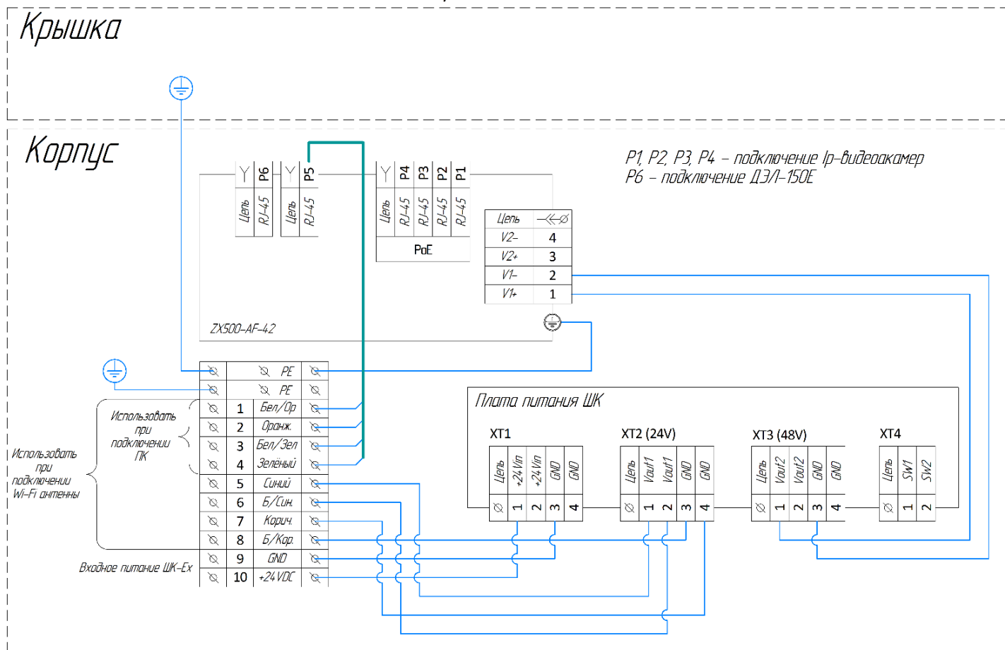
Рисунок 23. Схема электрическая соединений ШК-8-Ех
