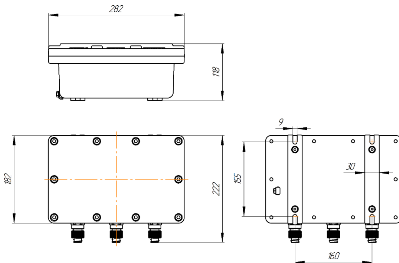
ПРИЛОЖЕНИЕ 7. Габаритный чертёж шкафа коммутации-1-ЕХ
