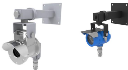
Рисунок 5. Видеокамера взрывозащищенная ВОВ-150
