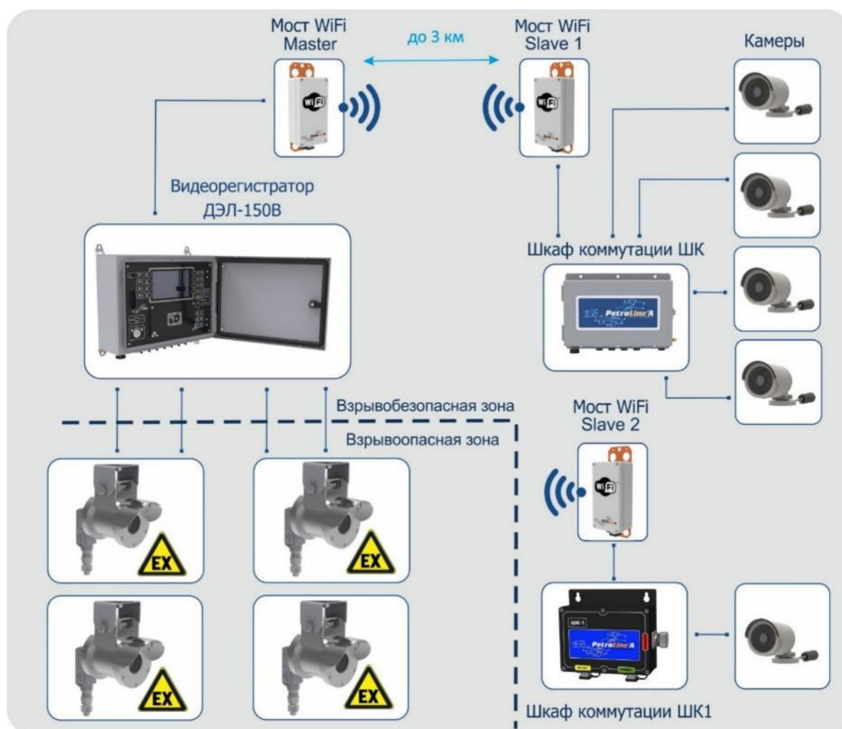
Рисунок 25. Пример №1 обобщенной блок-схемы подключения ДЭЛ-150ВЗ
