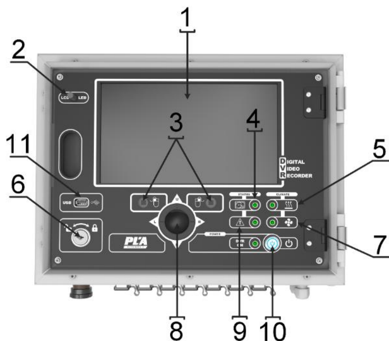
Рисунок 27. Лицевая панель видеорегистратора ДЭЛ-150В3-МДТ8
