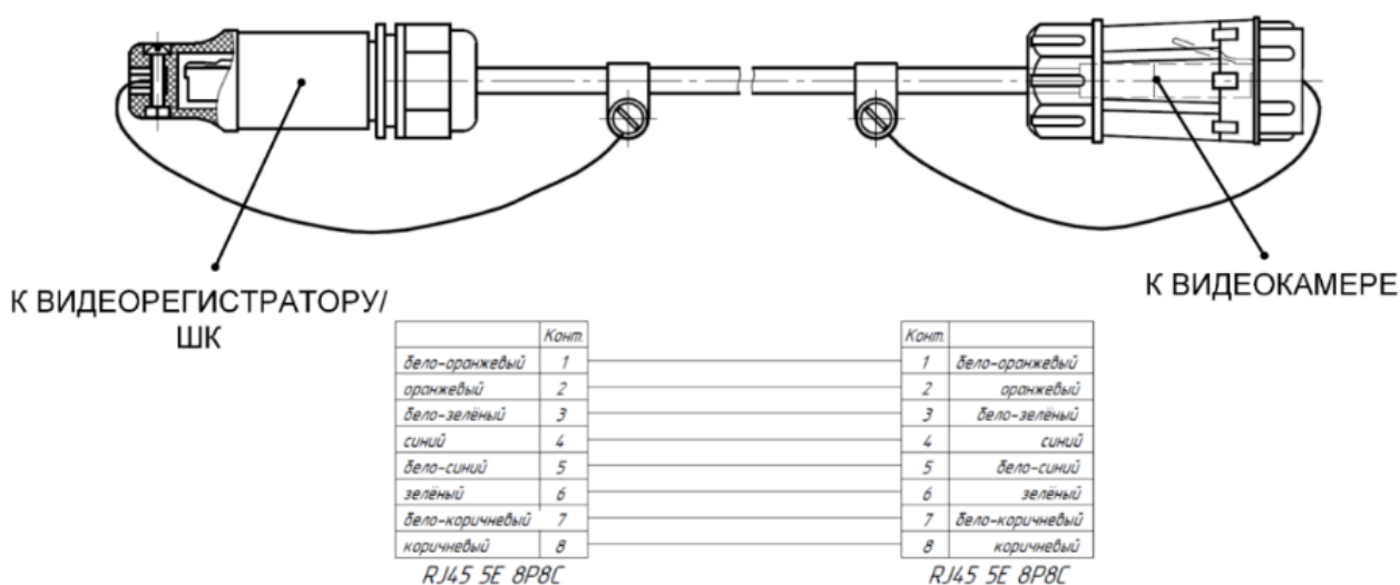
Рисунок 15. Кабель связи YUT-RJ/RJ45(муфта) для подключения камеры к видеорегистратору
