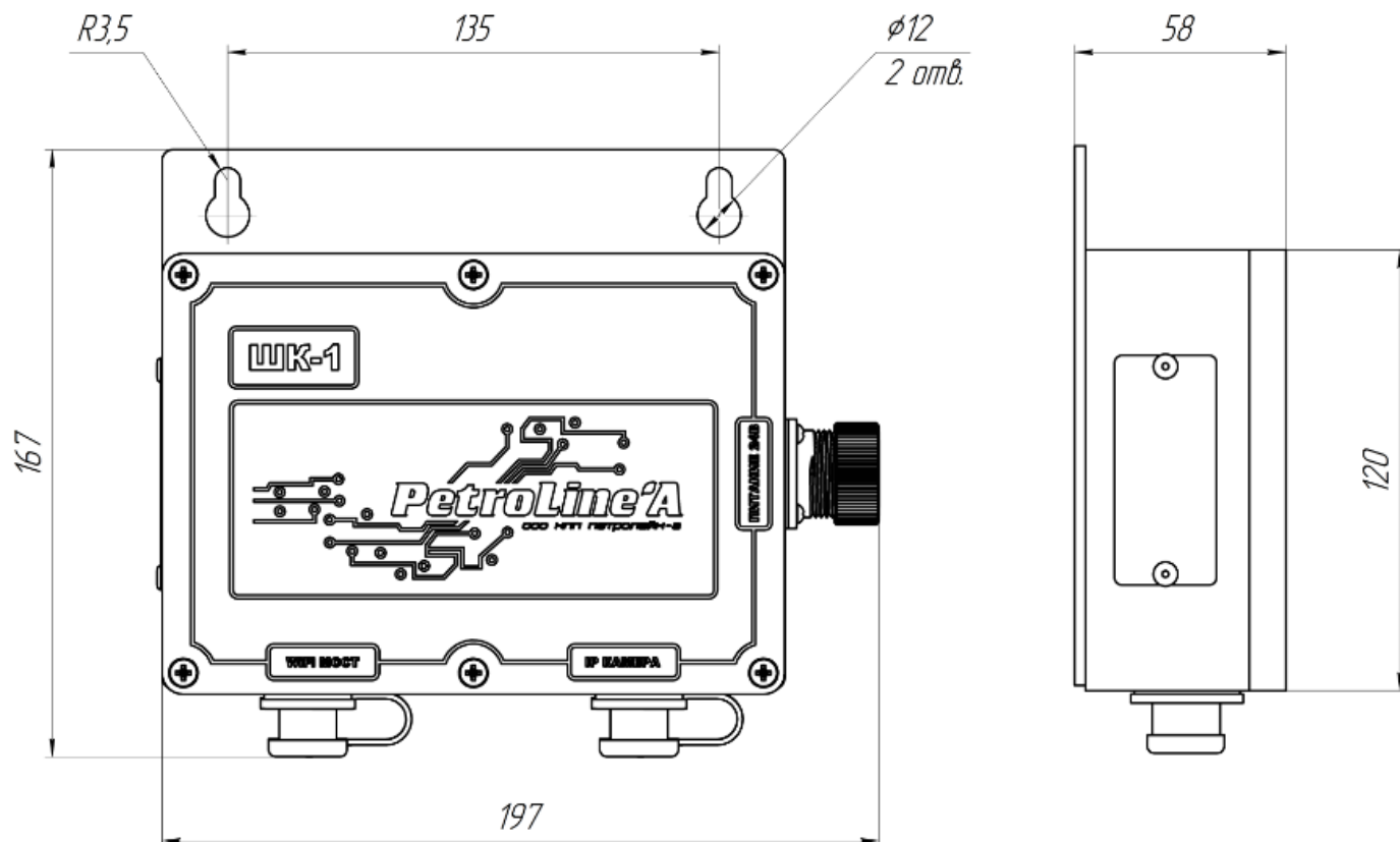
ПРИЛОЖЕНИЕ 6. Габаритный чертёж шкафа коммутации-1
