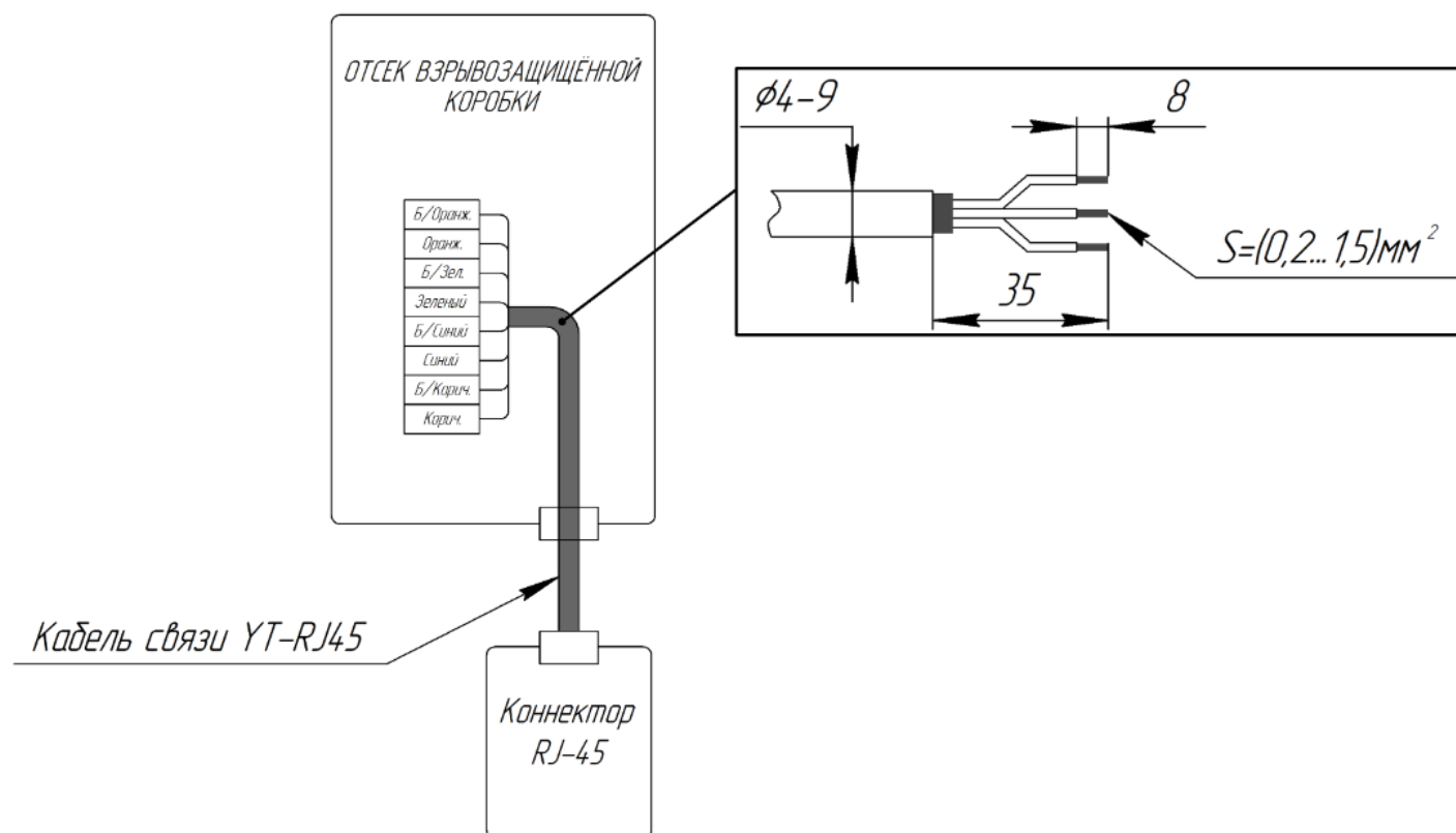
Рисунок 19. Схема подключения видеокамеры взрывозащищенной ВОВ-150
