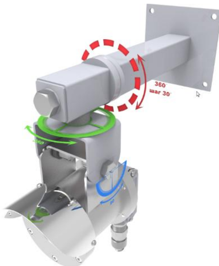
Рисунок 20. Угол поворота и наклона
