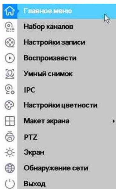
Рисунок 28. Контекстное меню
