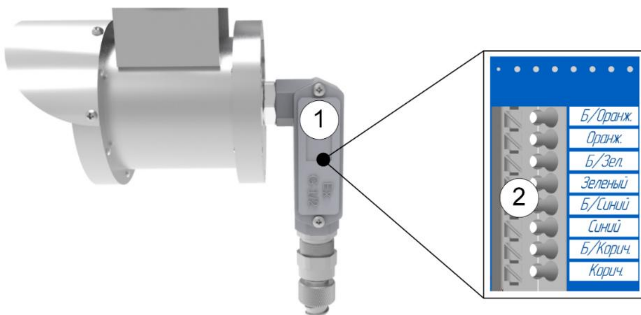
Рисунок 18. Отсек взрывозащищённой коробки
