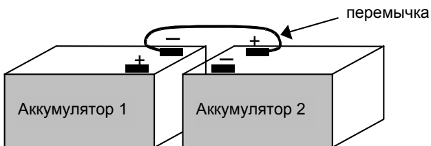
Рисунок 2. Схема соединения аккумуляторной батареи (АКБ)
