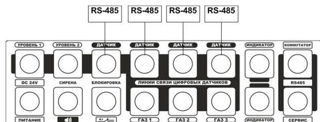
Кабель от У-150 подключается к любому из разъёмов МУ-150/МУ-150Е/МК-140 промаркированных «RS-485» (см. рисунок №10).
