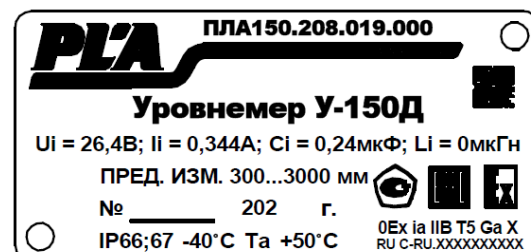
Рисунок 16. Пример маркировки У-150; У-150Д
