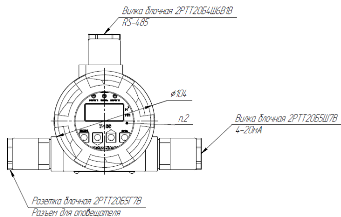
Рисунок 7. Габаритные и присоединительные размеры У-150Д
