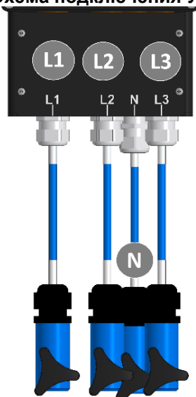
Рисунок 3. Схема подключения УНКСИ
