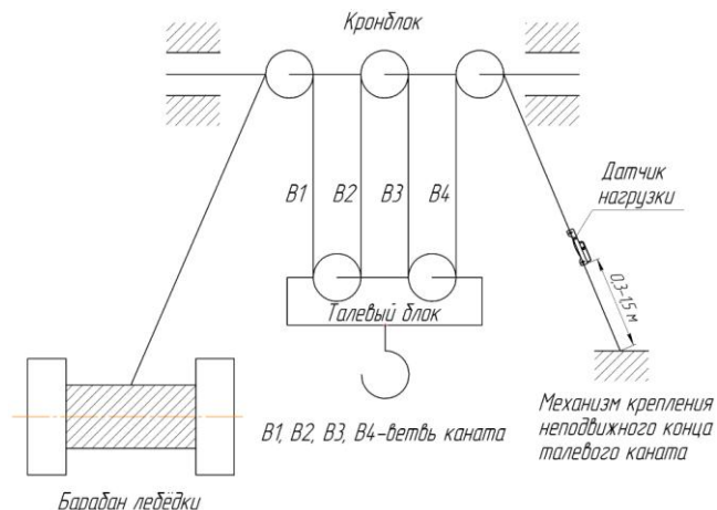
Рисунок 15. Схема талевой системы 2х3
